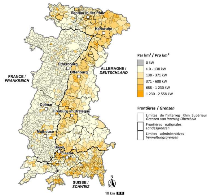
Puissance installée électrique du photovoltaïque dans le Rhin supérieur en 2024 Installierte elektrische Leistung von Photovoltaikanlagen im Oberrhein 2024
